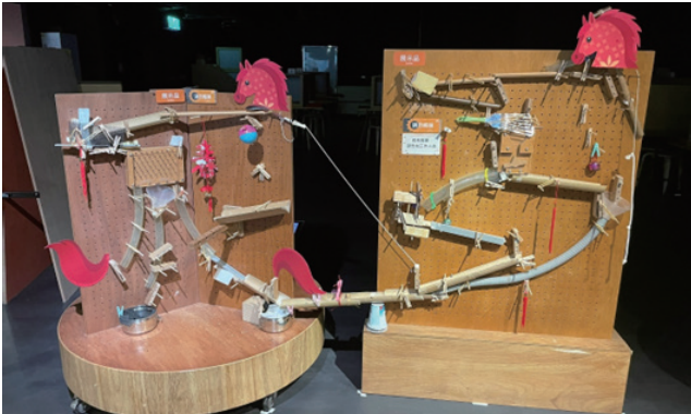
圖 1 彈珠機範例成品
